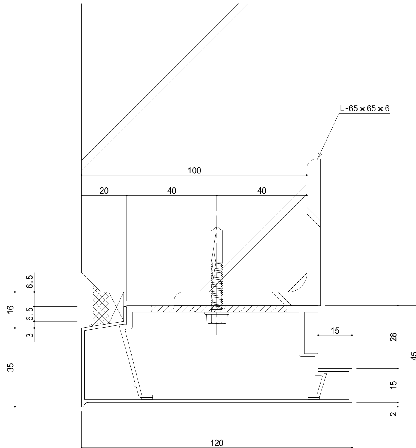
アルトップ 下端水切120 S = 1 / 1
