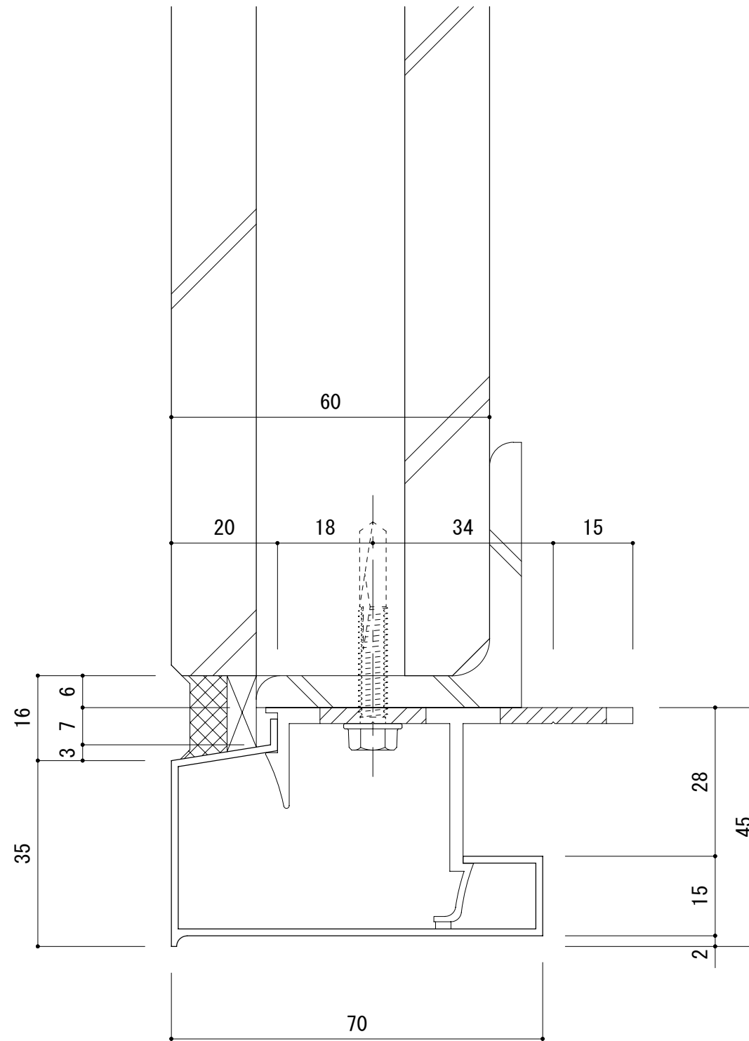
アルトップ 下端水切70 S=1/1
