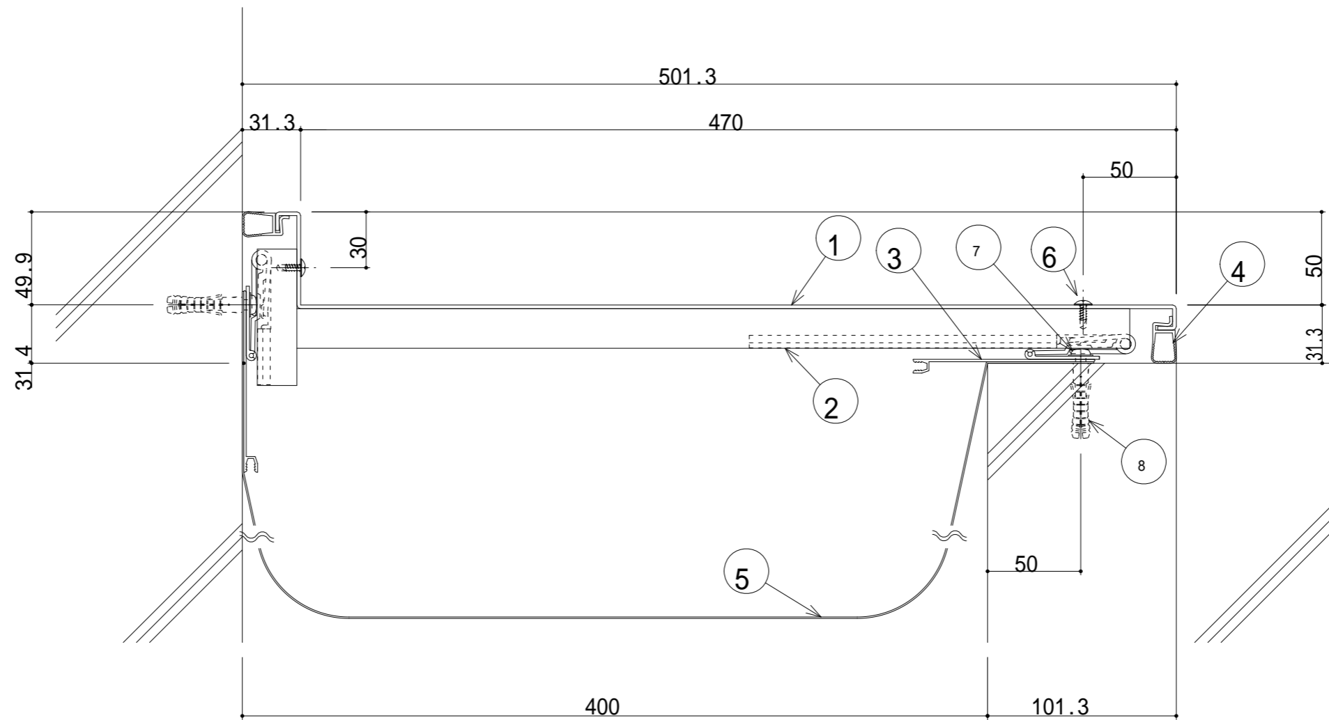
400-ECE 断面図
