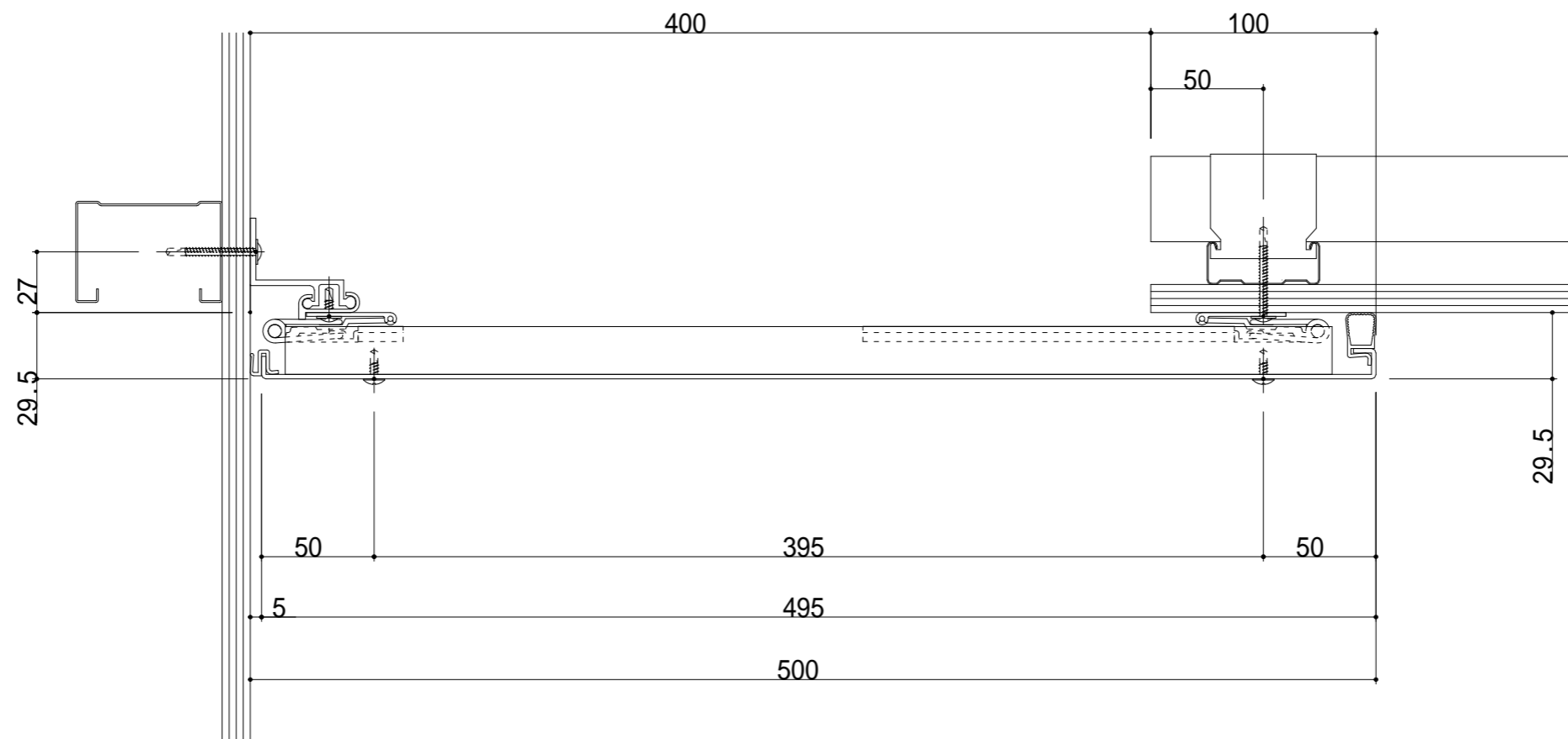
400-TCE 断面图
