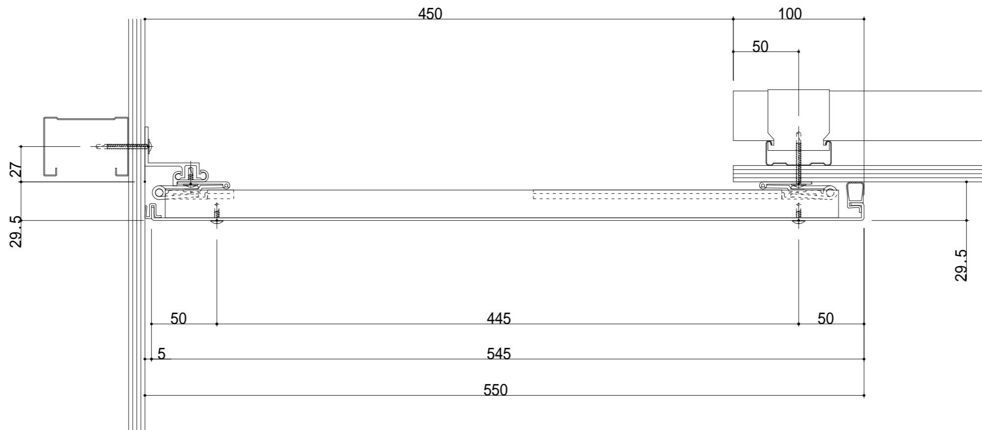
450-TCE 断面图
