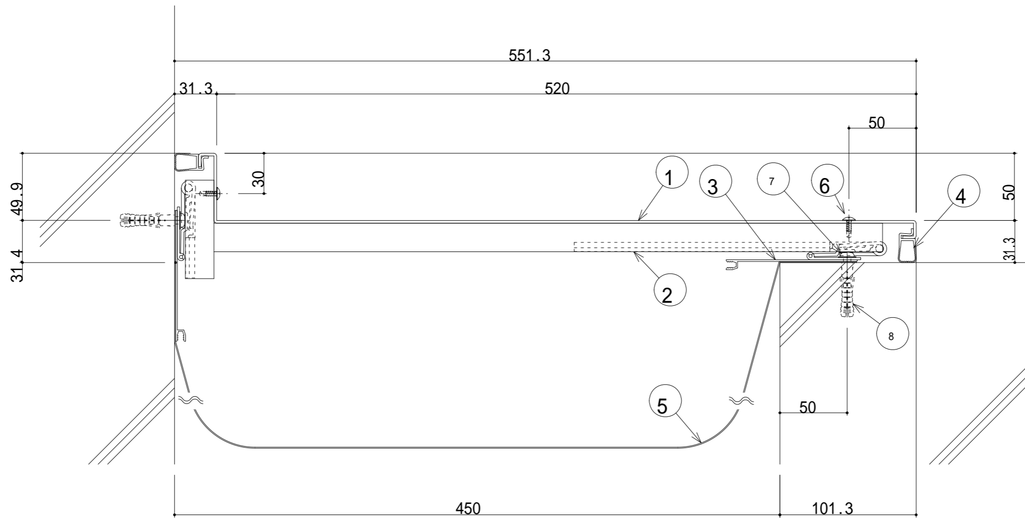
450-ECE 断面図
