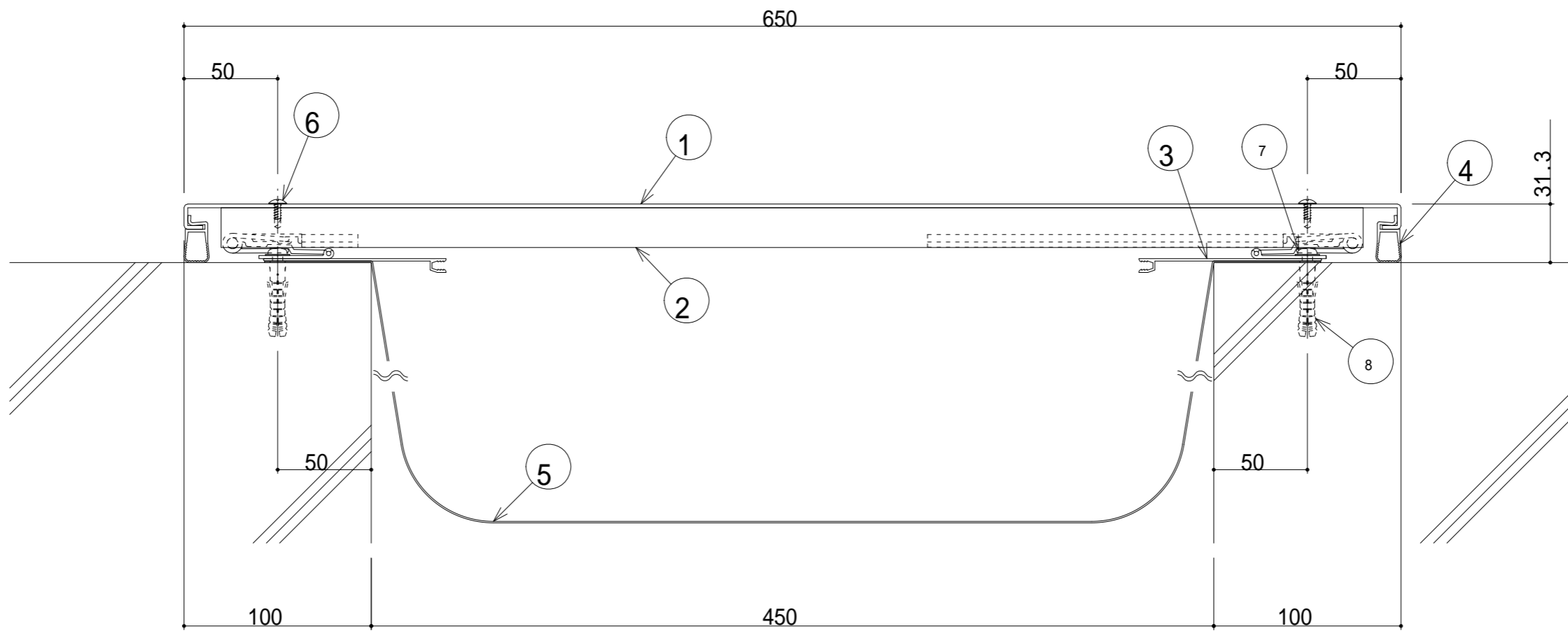
450-EE 断面図
