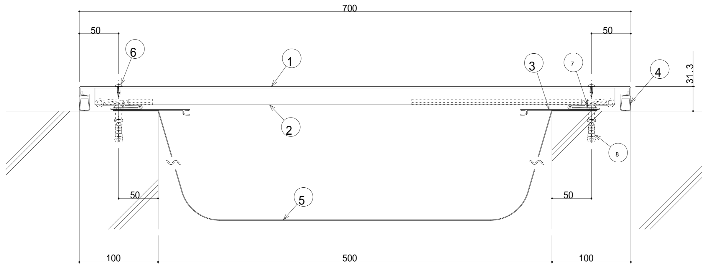
500-EE 断面図
