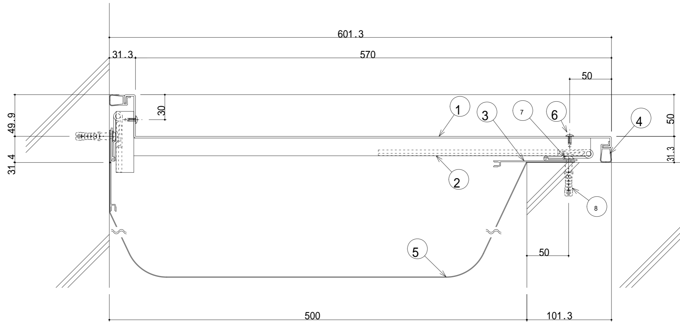
500-ECE 断面図
