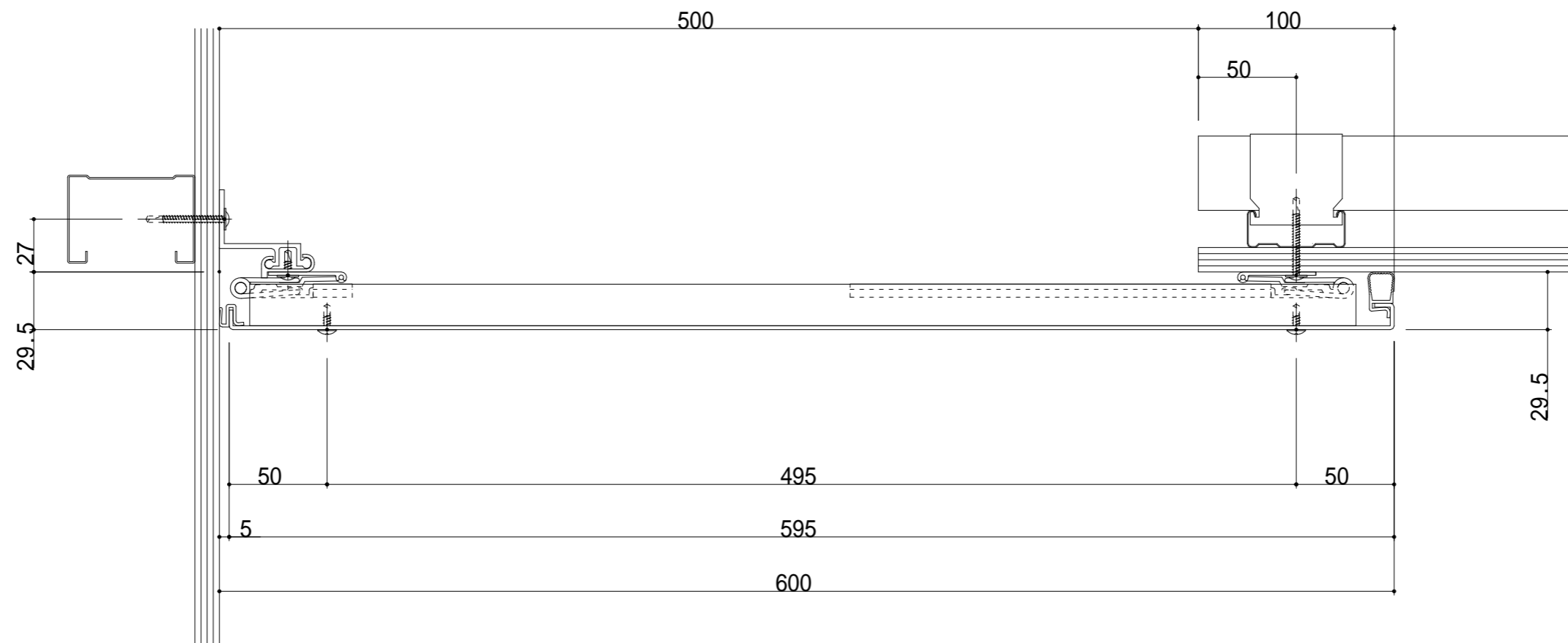
500-TCE 断面图
