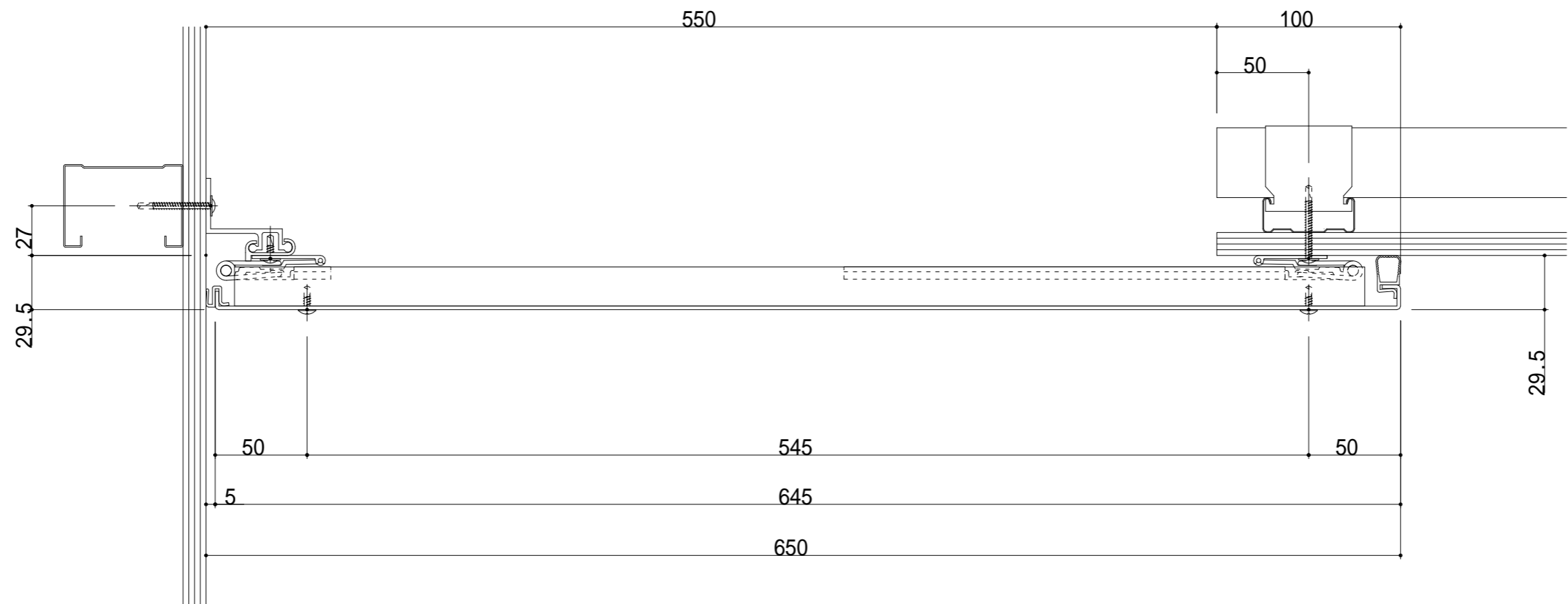
550-TCE 断面图
