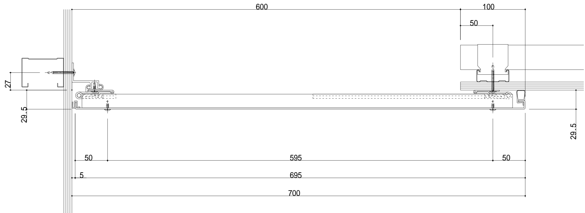
600-TCE 断面图
