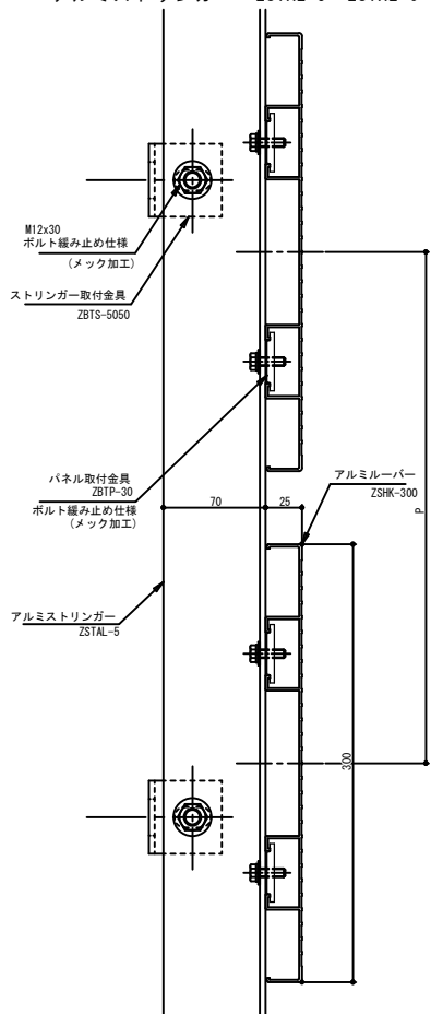
アルミストリンガー ZSTAL-5 ZSTAL-6
