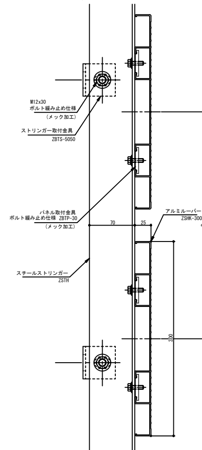
スチールストリンガー ZSTH
