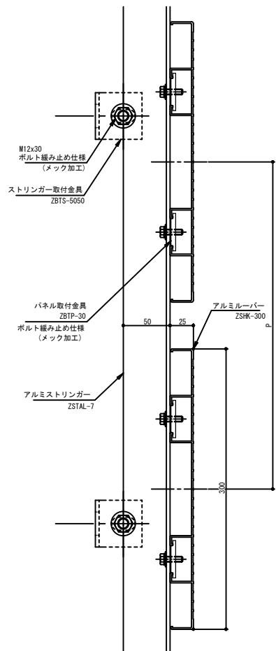
アルミルーバー ZSHK-300 アルミストリンガー ZSTAL-7 ZSTAL-8
