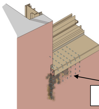
水が切れず水垂れ 汚れの原因に
