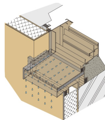
LLH 湿式外断熱システムの納まり
