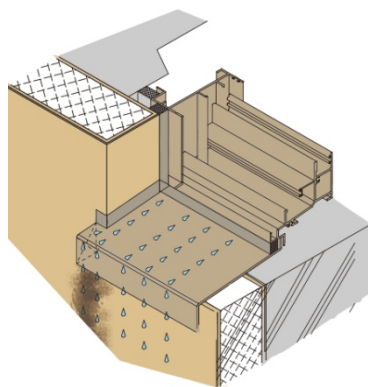
通常の湿式外断熱の納まり
