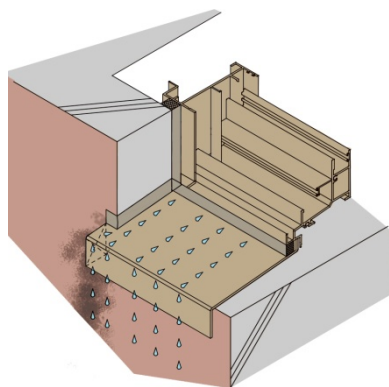
無断熱の納まり
